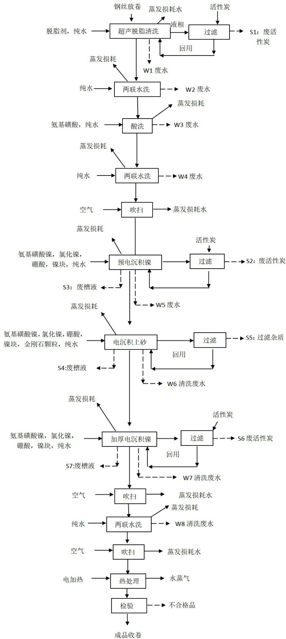
图 3.2-1 生产工艺流程图
