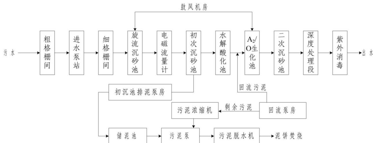
图 4.3-1 扬州市六圩污水处理厂污水处理工艺流程图
