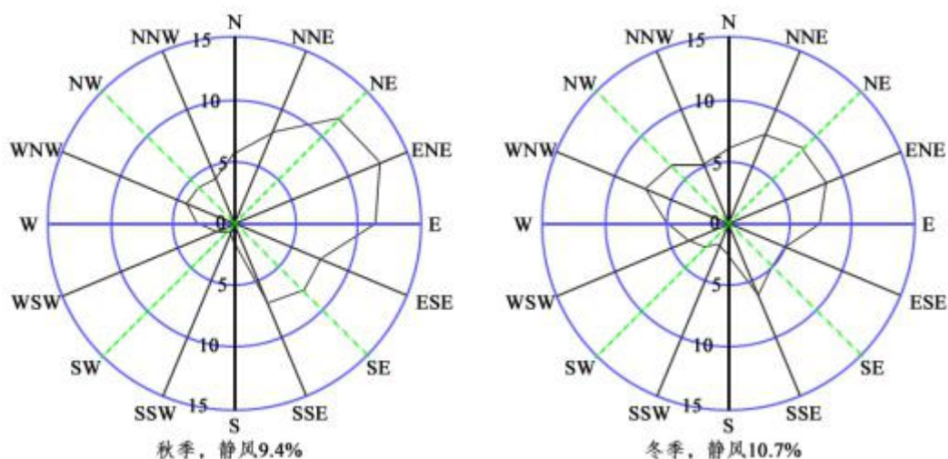
图 4.1-2 风频玫瑰图
