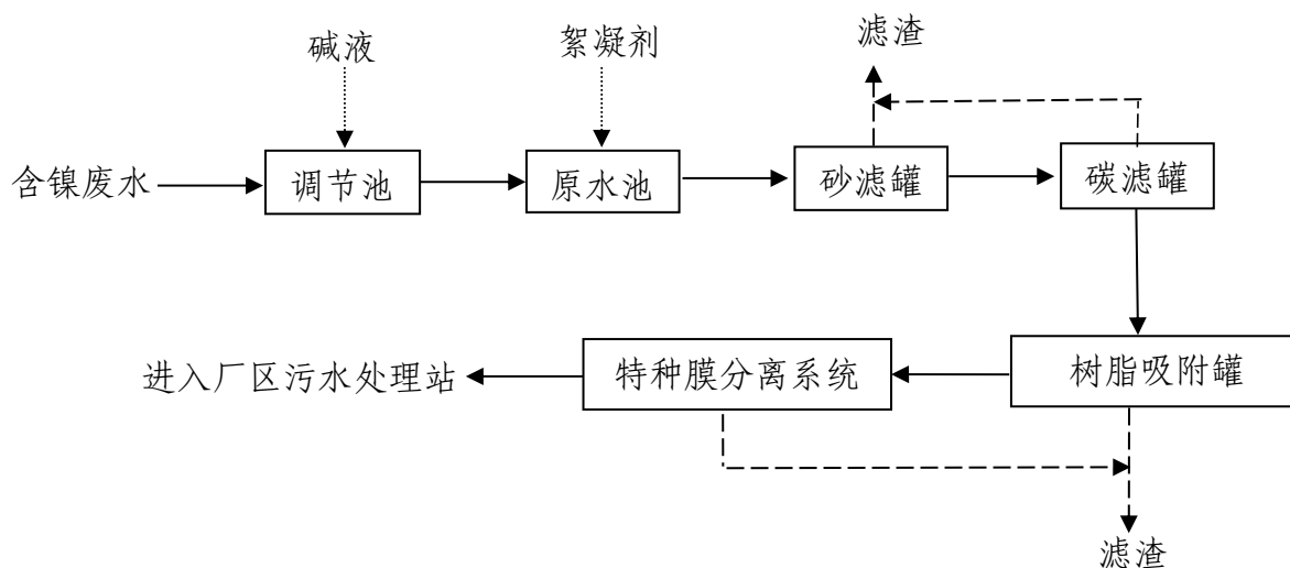
图 6.1-2 车间含镍废水预处理工艺图
