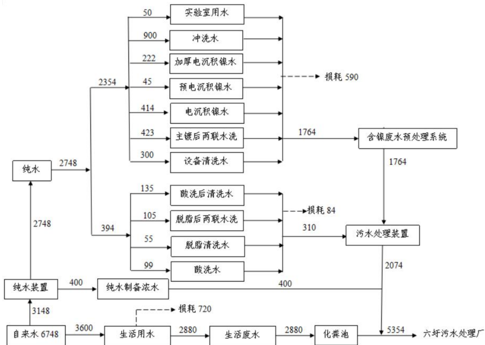
图 3.3-1 项目水平衡图 单位: \text{m}^3/\text{a}
