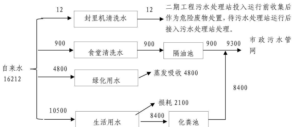
图 3.4-1 一期项目水平衡图 (m 3 /a)
